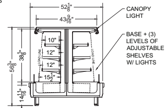
Section A:A View
